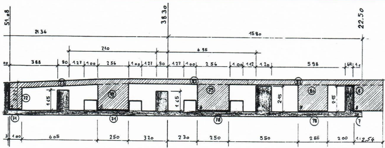
Schnitt durch Träger mit Deckenplatte zur Aufnahme weiterer Bauten. (Schraffierter Teil.)
